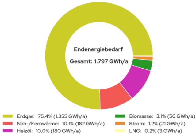
Abbildung 16: Endenergiebedarf nach Energieträger in Heilbronn
