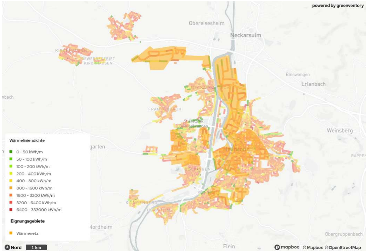
Abbildung 32: Wärmeliniendichte und resultierende Eignungsgebiete im Zieljahr
