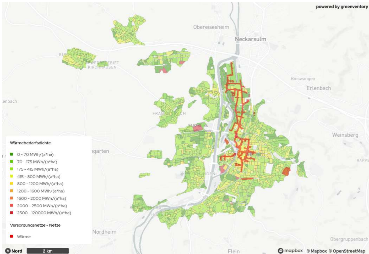
Abbildung 31: Wärmebedarfsdichte und bestehende Wärmenetze im Kerngebiet Heilbronn im Zieljahr
