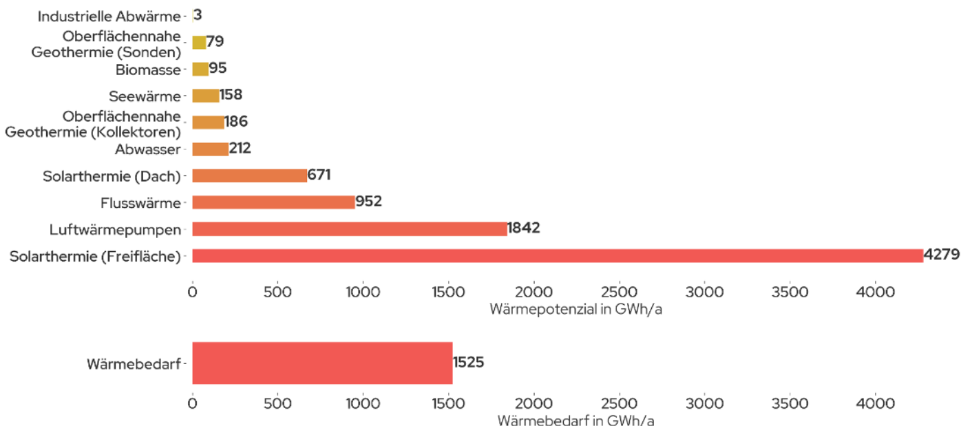
Abbildung 26: Erneuerbare Wärmepotenziale der Stadt Heilbronn
