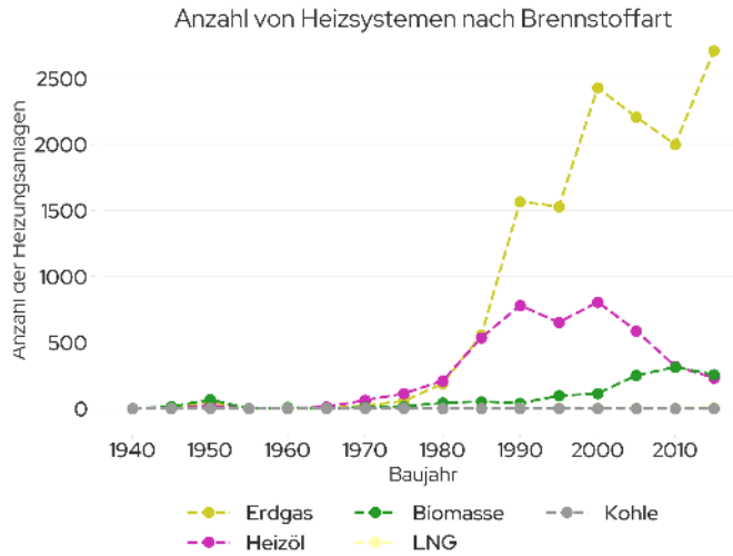
Abbildung 13: Verteilung der Anzahl der jährlich installierten Heizsysteme nach Baujahr und Energieträger
