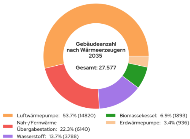
Abbildung 35: Gebäudeanzahl nach Wärmeerzeugern im Jahr 2035
