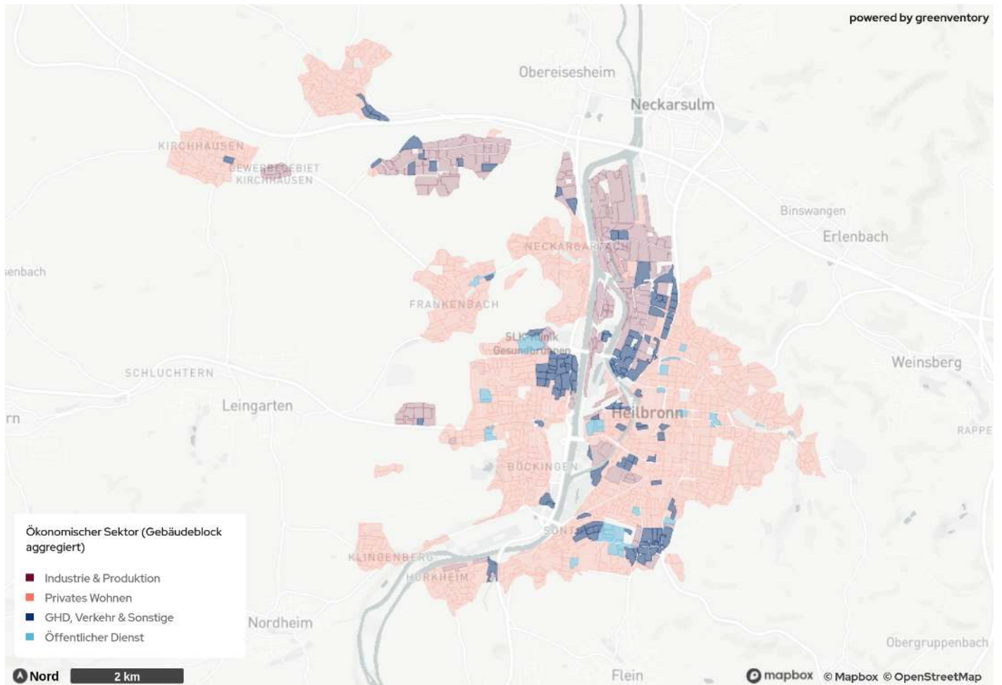
Abbildung 7: Verteilung der Gebäudezahl nach Sektor in Heilbronn
