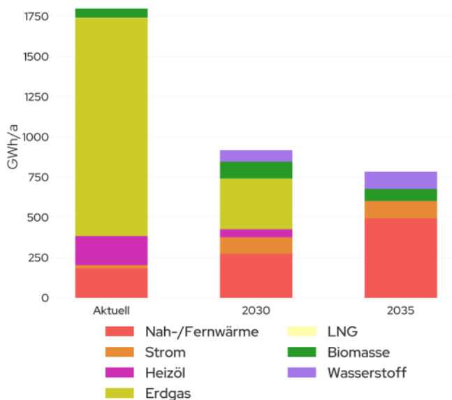
Abbildung 37: Verteilung des Endenergiebedarfs nach Energieträger im zeitlichen Verlauf
