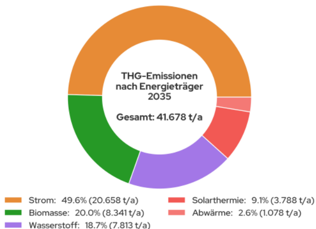
Abbildung 39: Treibhausgas-Emissionen nach Energieträger im Jahr 2035
