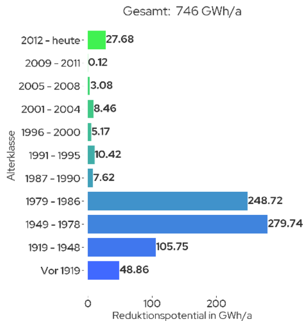
Abbildung 27: Reduktionspotential nach Baualterklassen
