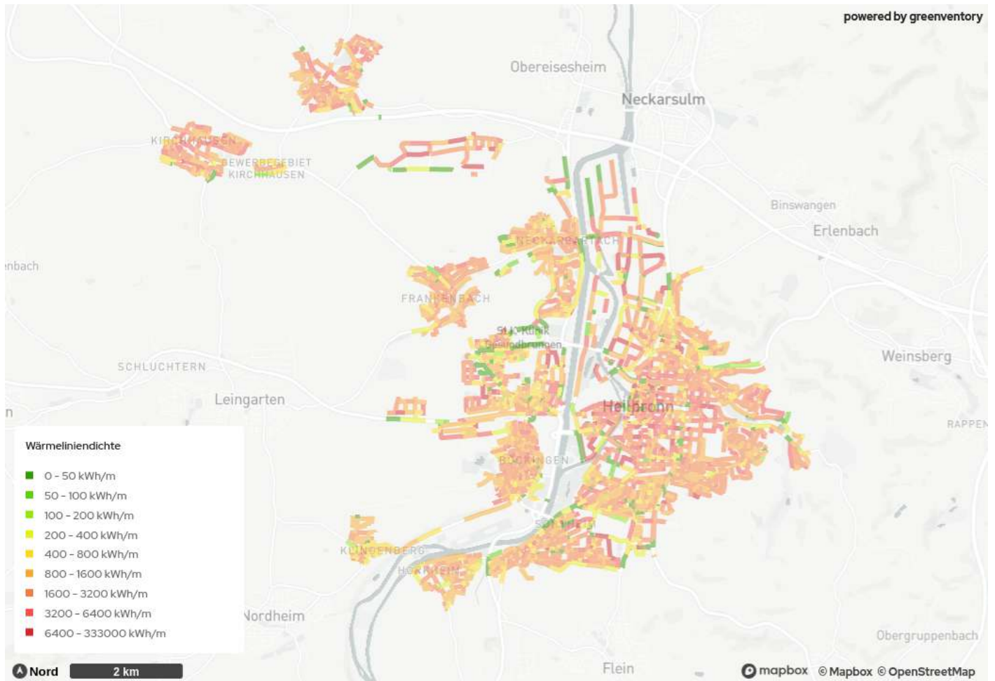
Abbildung 30: Wärmeliendichte im Kerngebiet Heilbronn im Zieljahr
