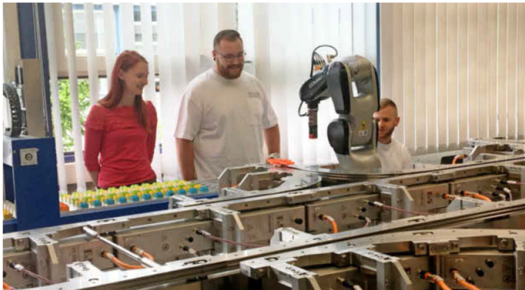
Praxisnahe - Schüler der Wilhelm Maybach Schule haben für die Lernfabrik 4.0 als Technikerarbeit eine Roboterzelle mit 6-Achs-Roboter aufgebaut und in Betrieb genommen. Foto: Markus Sütterlin
